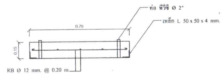
รูปตัดฝายบ่อบำบัดน้ำ จุดที่ 3 NOT to scale
