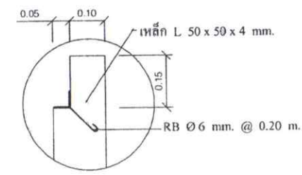
รูปขยาย จุดที่ 3 NOT to scale
